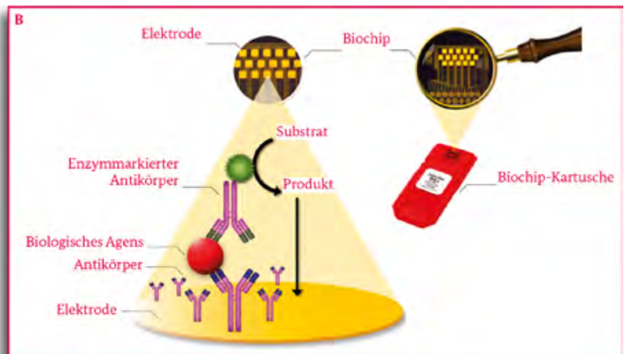
Abbildung 1: Die Biochip-basierte pTDi-Plattform der Bruker Daltonik GmbH. (A) Tragbare pTDi-Plattform (Prototyp) zum Vor-Ort-Nachweis biologischer Agenzien. (B) Darstellung des elektronischen Biochips in der Biochip-Kartusche sowie das Detektionsprinzip.
